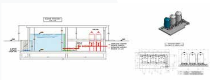
Planimetria e sezione tipologica dell’impianto di filtrazione GAC.
